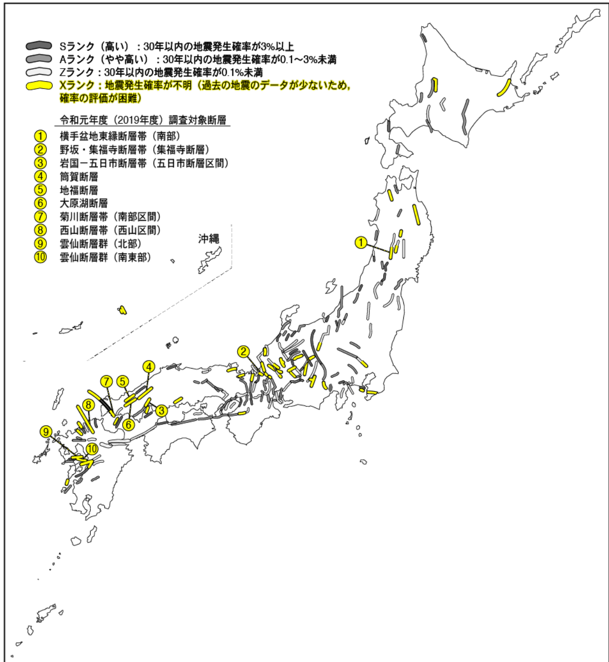
図1 将来の地震発生確率によりランク分けされた全国主要活断層の分布と令和元年度調査対象の10断層 (区間) (地震調査研究推進本部, 2020, 「主要活断層の評価」 https://www.jishin.go.jp/evaluation/evaluation_summary/#danso (2020年3月31日閲覧) を編集)。
