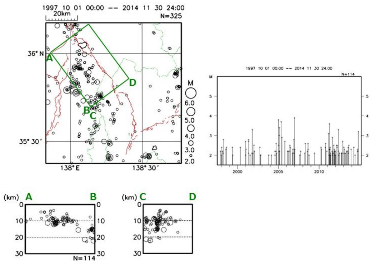
図 8－6 中南部（諏訪湖北方～下葛木）区間の地震活動（震源データは図 8－1 同様） 1997 年 10 月 1 日～2014 年 11 月 30 日（M2.0 以上、深さ 30km 以浅）
