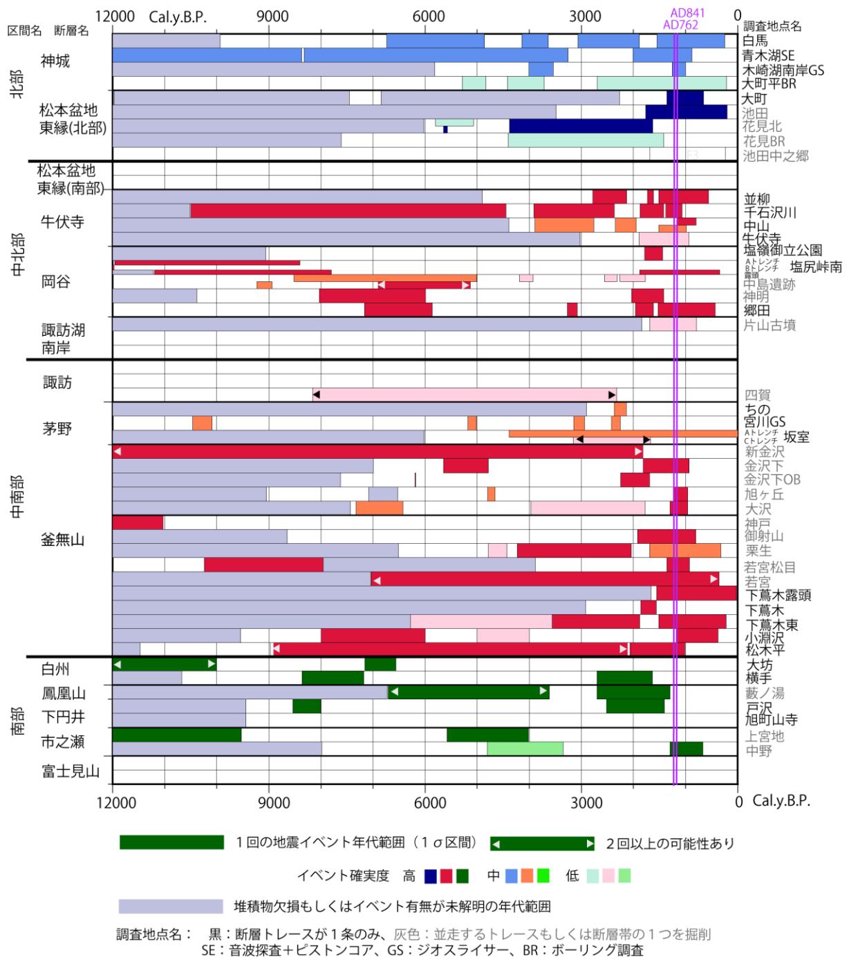
図6-1 本断層帯の最近約1万2千年間の地震イベントダイアグラム(文部科学省研究開発局ほか(2010)の結果に郷田(近藤・谷口, 2014)を追加)
