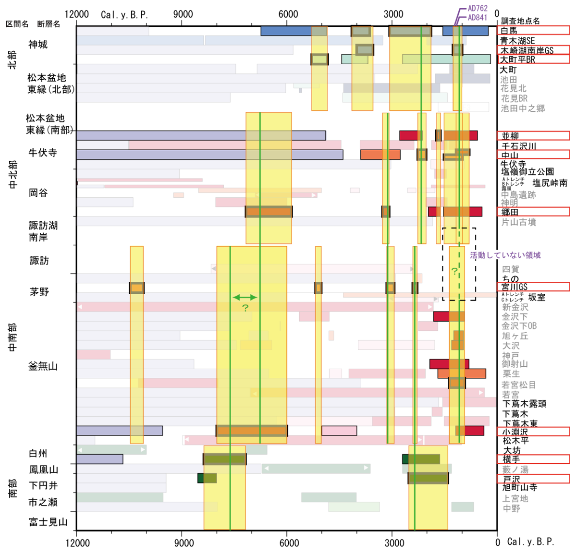
図6-2 本断層帯の最近約1万2千年間の地震イベントの解釈図（黄矩形）
