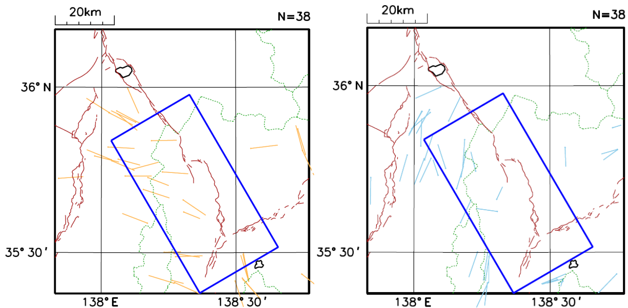
図 8 - 9 図 8 - 8 の領域内の発震機構の圧力軸（左）と張力軸（右）の分布 1997 年 10 月 1 日～2014 年 11 月 30 日（深さ 30km 以浅）
