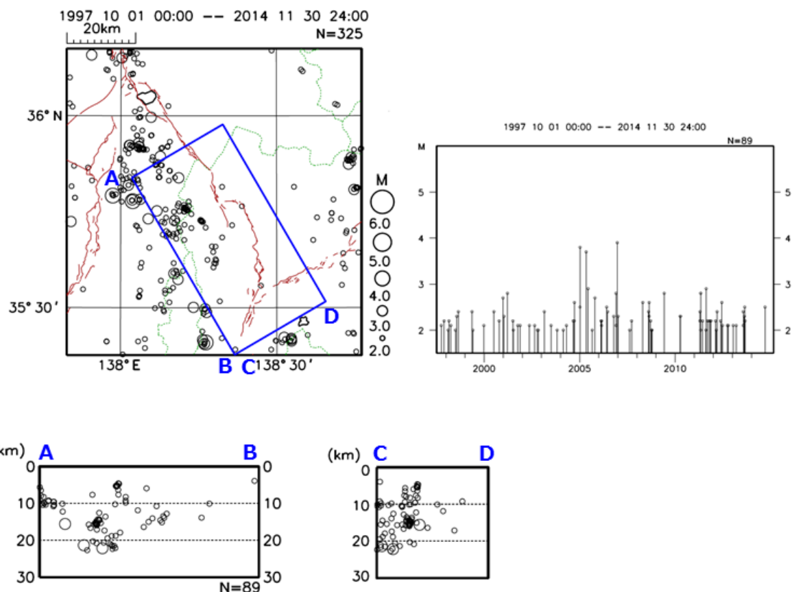
図 8 - 8 南部（白州－富士見山）区間の地震活動（震源データは図 8 - 1 同様） 1997 年 10 月 1 日～2014 年 11 月 30 日（M2.0 以上、深さ 30km 以浅）
