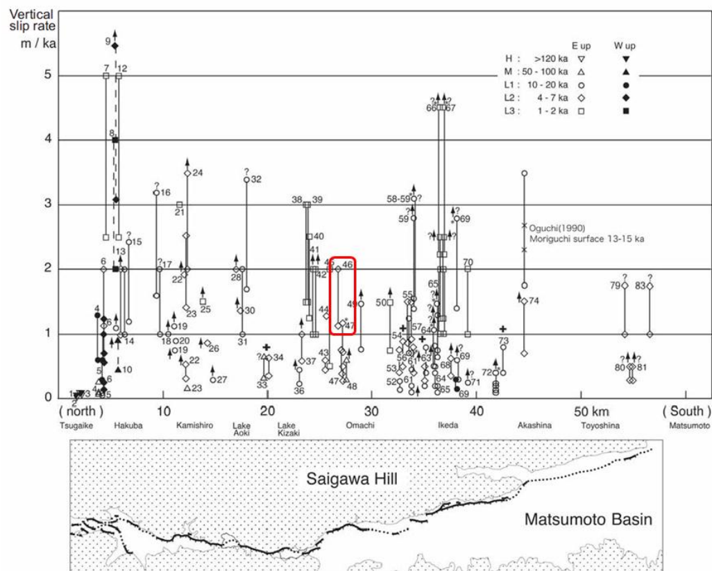
図5－1 北部(小谷－明科)区間の平均変位速度分布(上下) (文部科学省研究開発局ほか, 2010)。 赤枠は評価に用いられたデータを示す。
