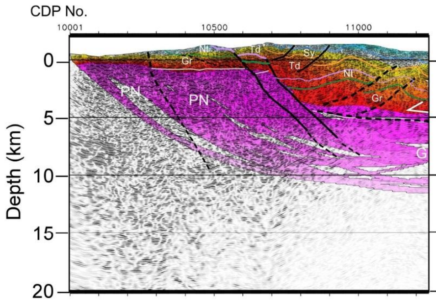
図 4-1 飯山ー小谷測線（図 2- 1 の測線 A）に沿う反射法弾性波探査断面、屈折トモグラフィとその地質学的解釈による小谷ー中山断層（CDP10700 付近の地表から 11000 の 5-10km 深に向かって傾斜する実線）（佐藤ほか，2012）
