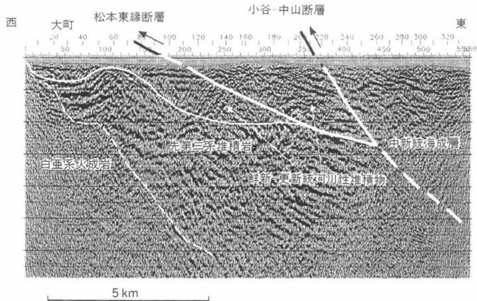
図 4-2 松本盆地東縁断層北半部から長野盆地に向かう測線（図 2- 1 の測線 B）に沿う反射法弾性波探査断面とその解釈（佐藤・平田，1998）
