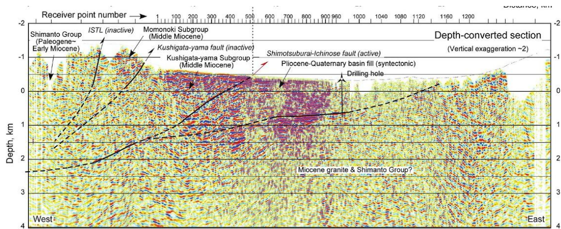
図 4-5 御勅使川沿いの反射法地震探査（図 2-4 の測線 H）による深度断面図（池田ほか，2009）
