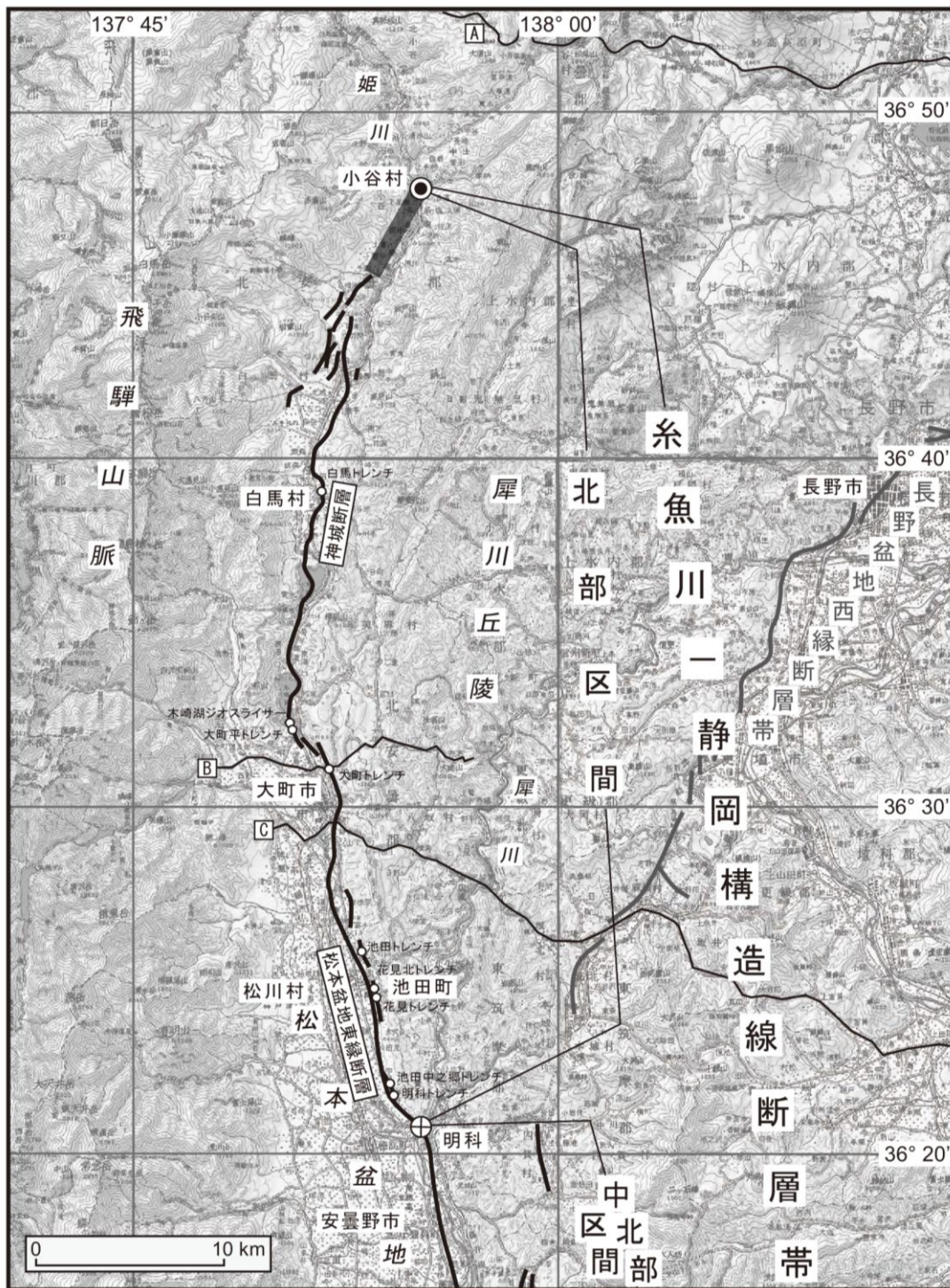
図 2-1 糸魚川—静岡構造線断層帯北部（小谷—明科）区間の活断層位置
