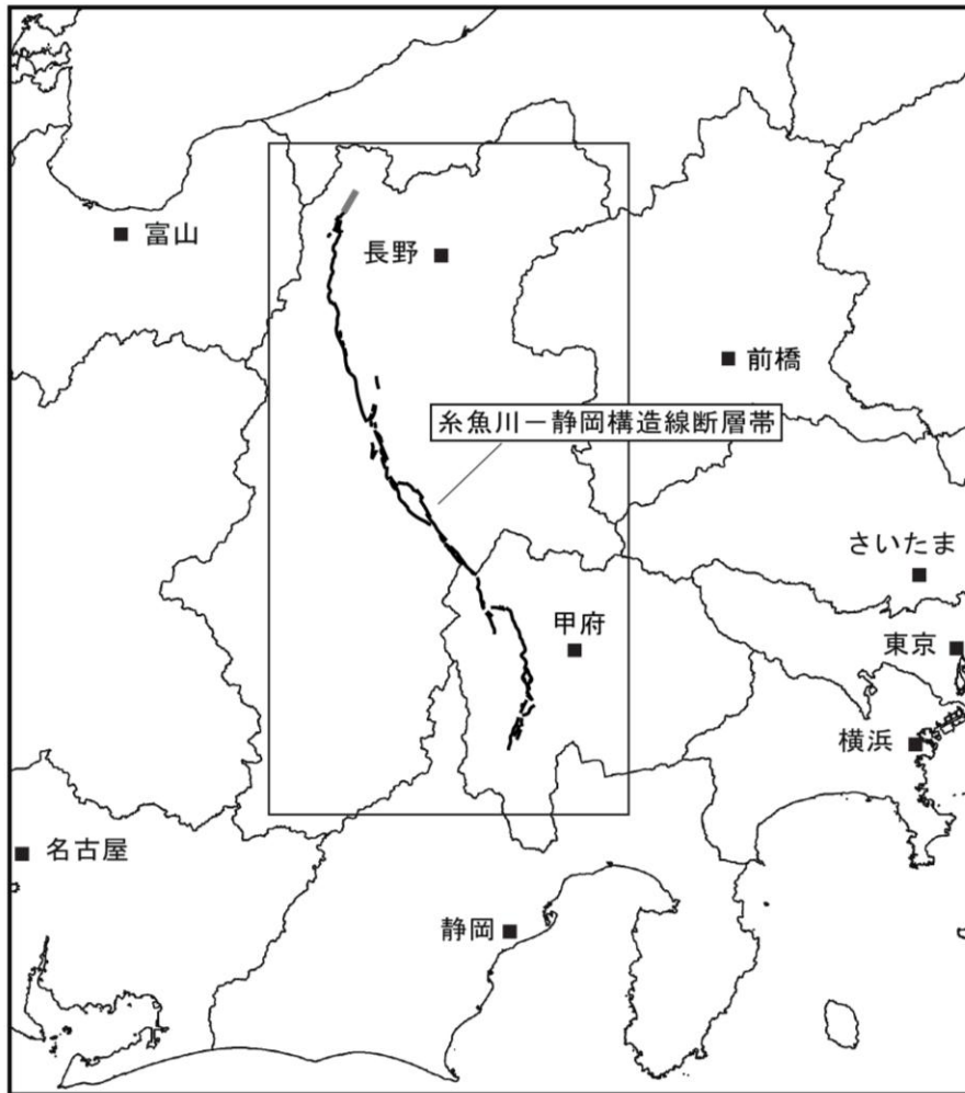
図 1 - 1 糸魚川—静岡構造線断層帯の概略位置図 (長方形は図 1 - 2 の範囲)
