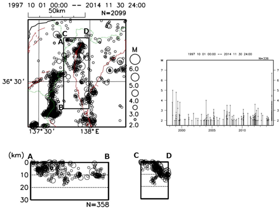
図 8 - 2 北部（小谷－明科）区間の地震活動
