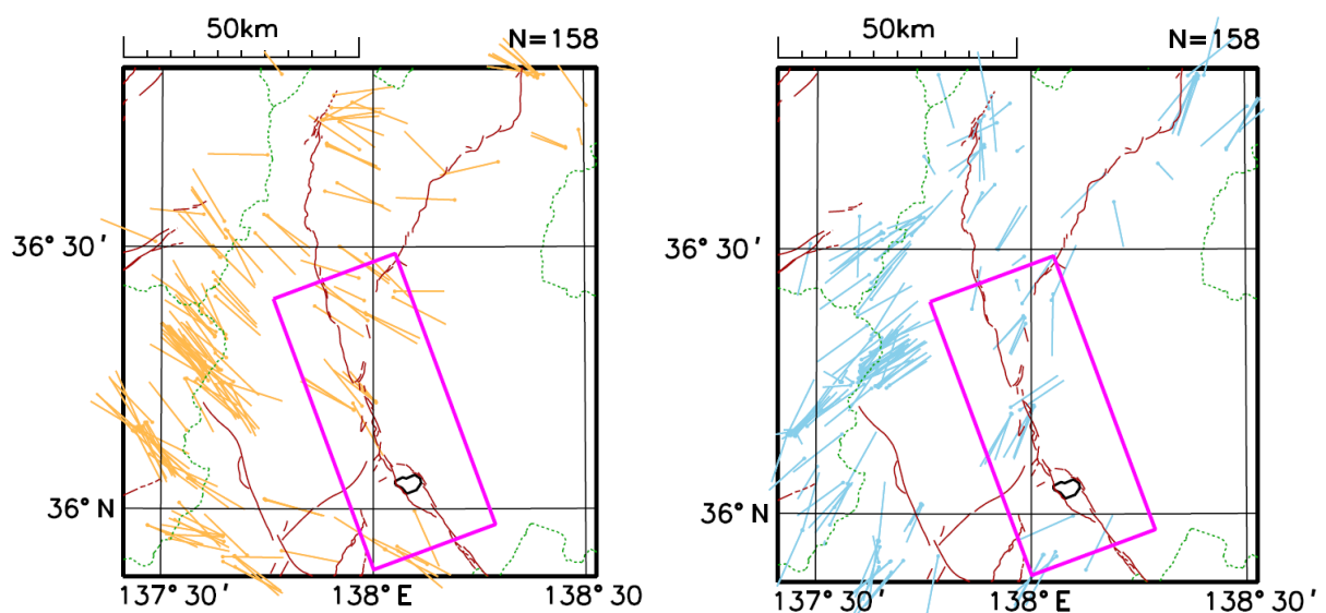
図 8 - 5 図 8 - 4 の領域内の発震機構の圧力軸（左）と張力軸（右）の分布 1997 年 10 月 1 日～2014 年 11 月 30 日（深さ 30km 以浅）
