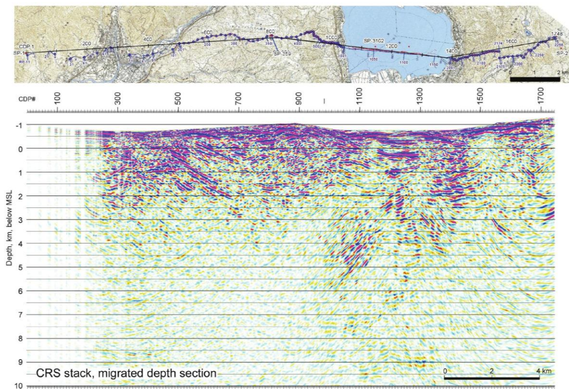
図4-3 測線E（図2-2）に沿う反射法地震探査結果（池田ほか，2009）
