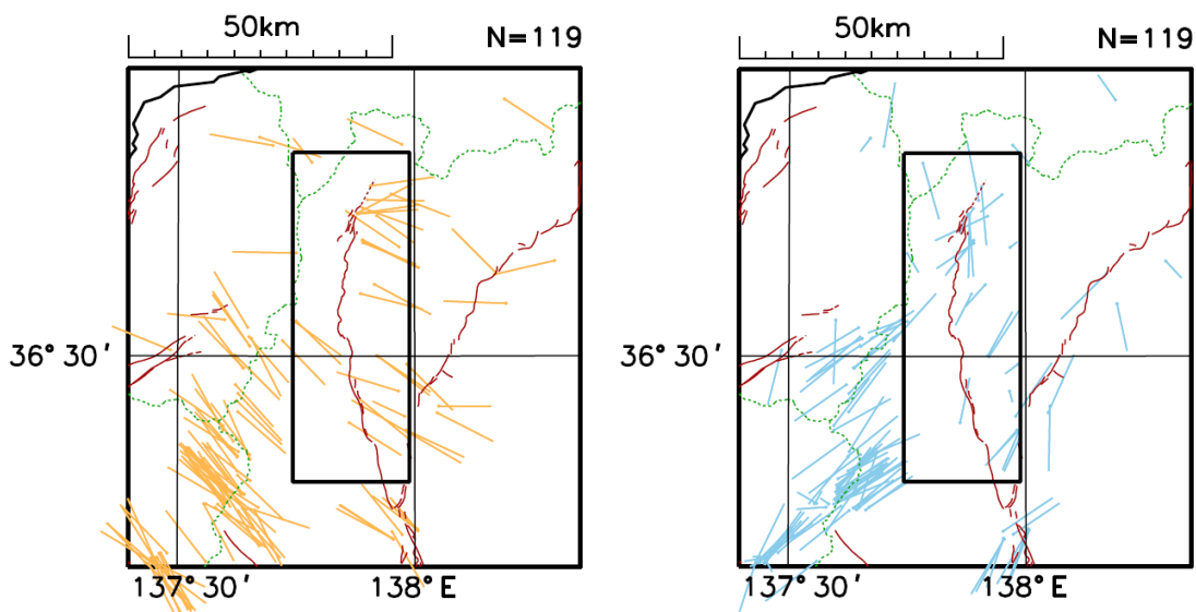
図 8 - 3 図 8 - 2 の領域内の発震機構の圧力軸（左）と張力軸（右）の分布
