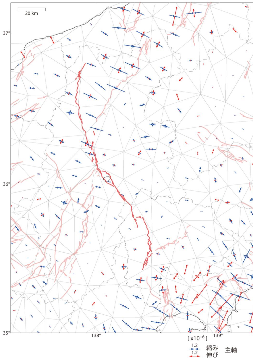
図 7-1 2004 年 11 月から 2011 年 2 月までの GNSS 連続観測による糸魚川－静岡構造線断層帯周辺の水平ひずみ速度分布（国土地理院作成）
