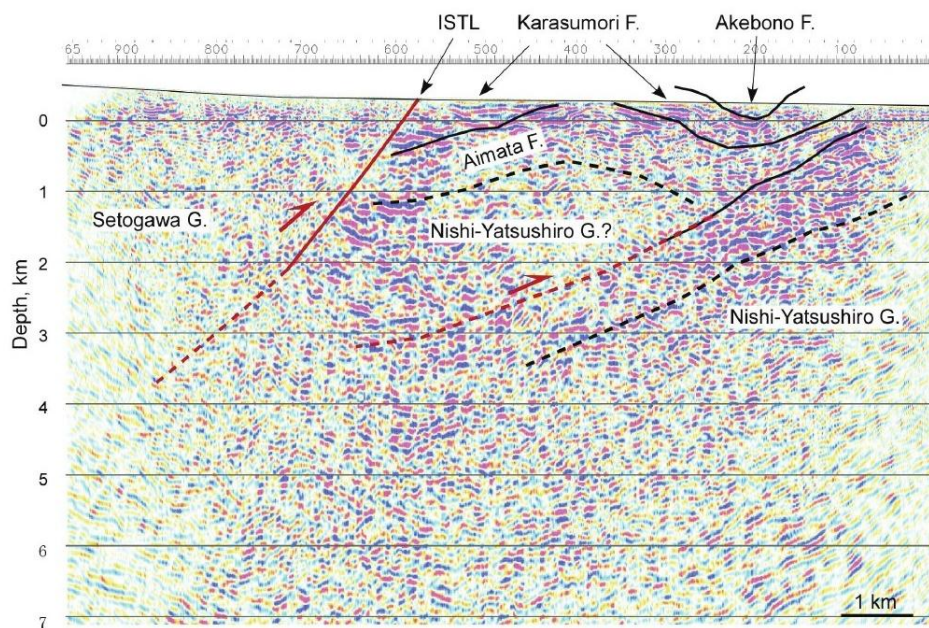
図 4-6 反射法地震探査（図 2 の測線 I）による深度断面及びその解釈（池田ほか，2009）
