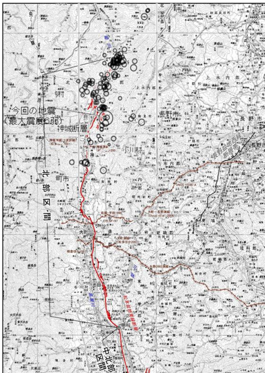
図3 本断層帯北部（小谷－明科）区間のトレースと2014年11月22日に発生した地震（M6.7）の本震及び余震分布（震源分布は気象庁の平成26年11月23日11時55分の報道発表資料）
