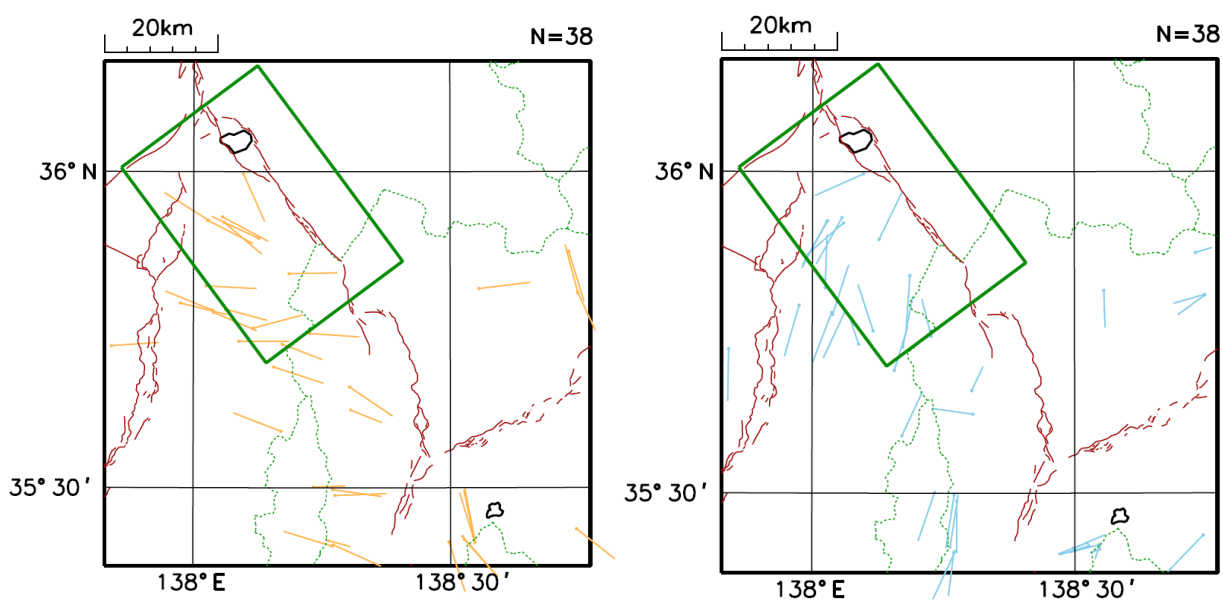
図 8－7 図 8－6 の領域内の発震機構の圧力軸（左）と張力軸（右）の分布 1997 年 10 月 1 日～2014 年 11 月 30 日（深さ 30km 以浅）
