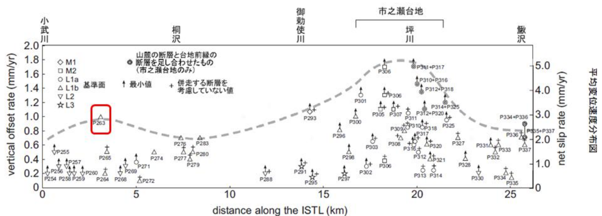
図 5-4 南部（白州－富士見山）区間（下円井断層、市之瀬断層群）の平均変位速度分布（上下） （文部科学省研究開発局ほか, 2010）。
