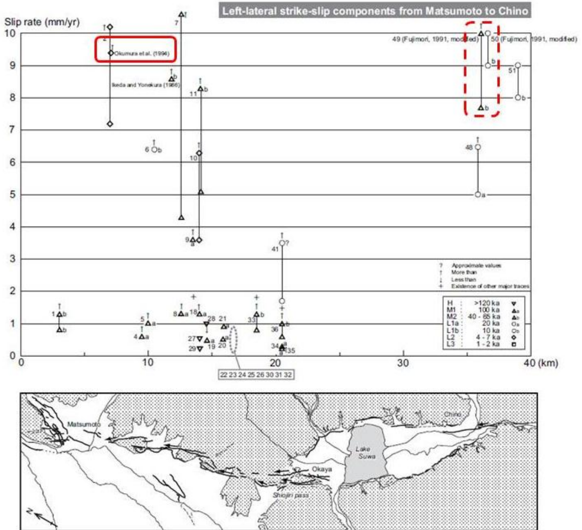
図5-2 中北部（明科－諏訪湖南方）区間及び中南部（諏訪湖北方－下葛木）区間の平均変位速度分布（左横ずれ）（文部科学省研究開発局ほか, 2010）。 中北部区間の赤枠（左）は評価に用いられたデータ、中南部区間の赤枠（右の点線）は検討に用いられたデータを示す。
