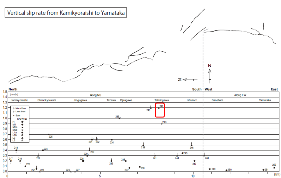
図 5-3 南部（白州－富士見山）区間（白州断層、鳳凰山断層）の平均変位速度分布（上下） （文部科学省研究開発局ほか, 2010）。
