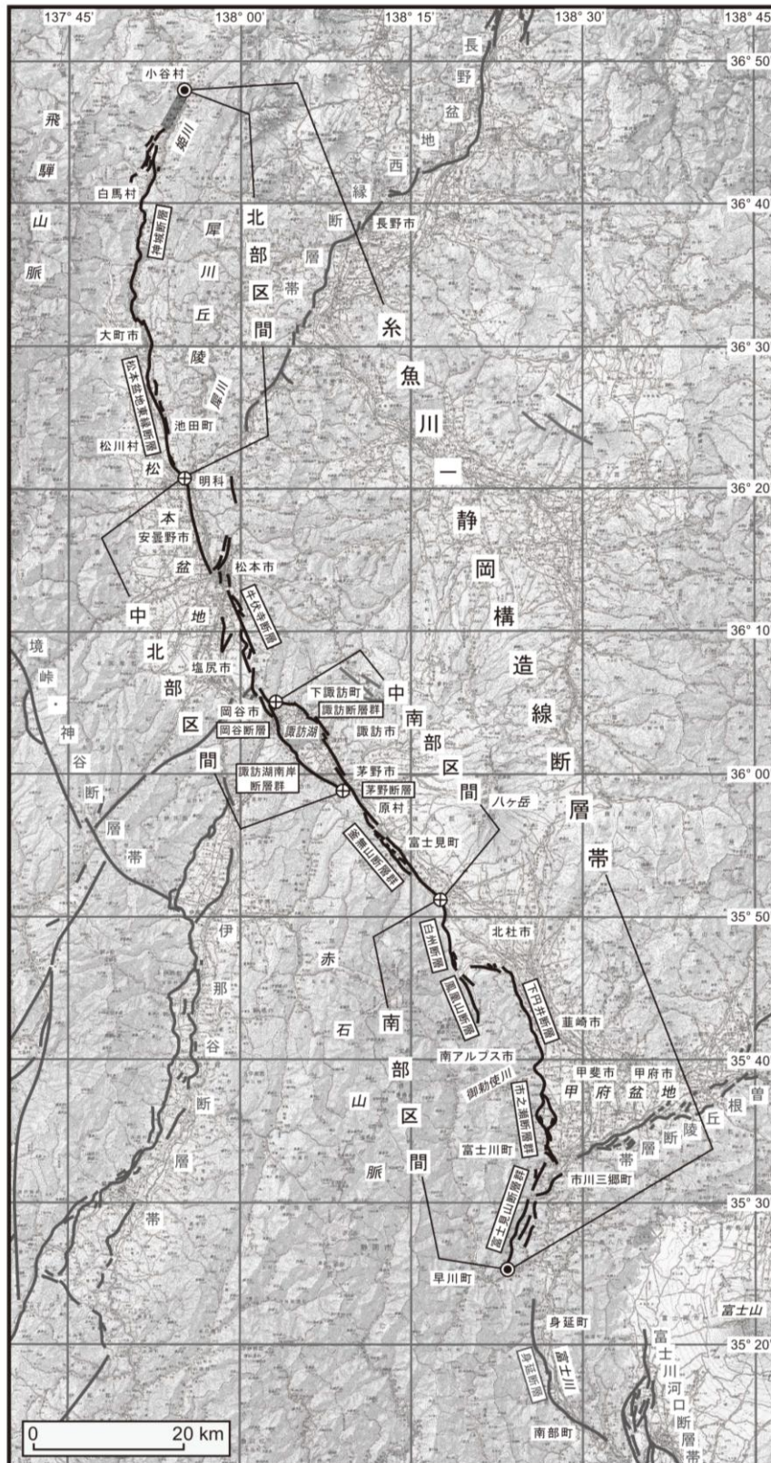
図 1-2 糸魚川—静岡構造線断層帯の活動区間
