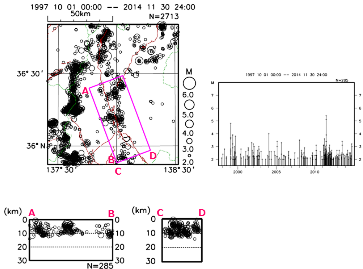
図 8 - 4 中北部（明科－諏訪湖南方）区間の地震活動（震源データは図 8 - 1 同様） 1997 年 10 月 1 日～2014 年 11 月 30 日（M2.0 以上、深さ 30km 以浅）
