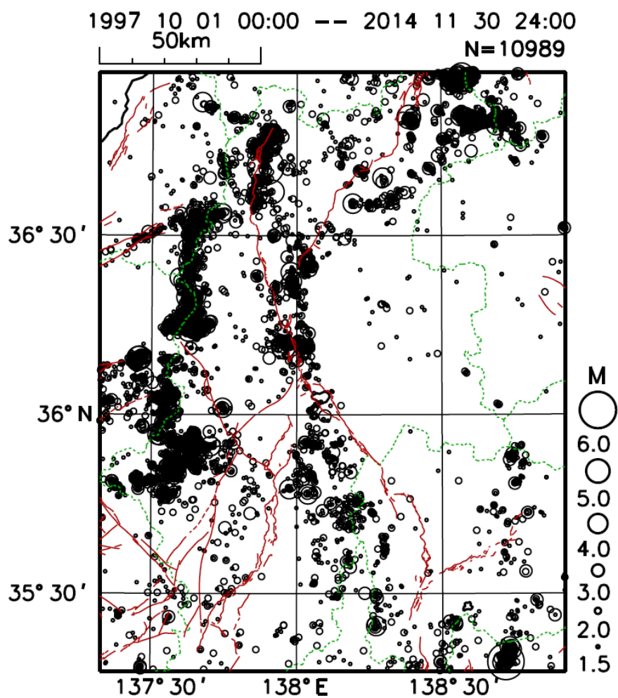
図 8 - 1 本断層帯周辺の地震活動
