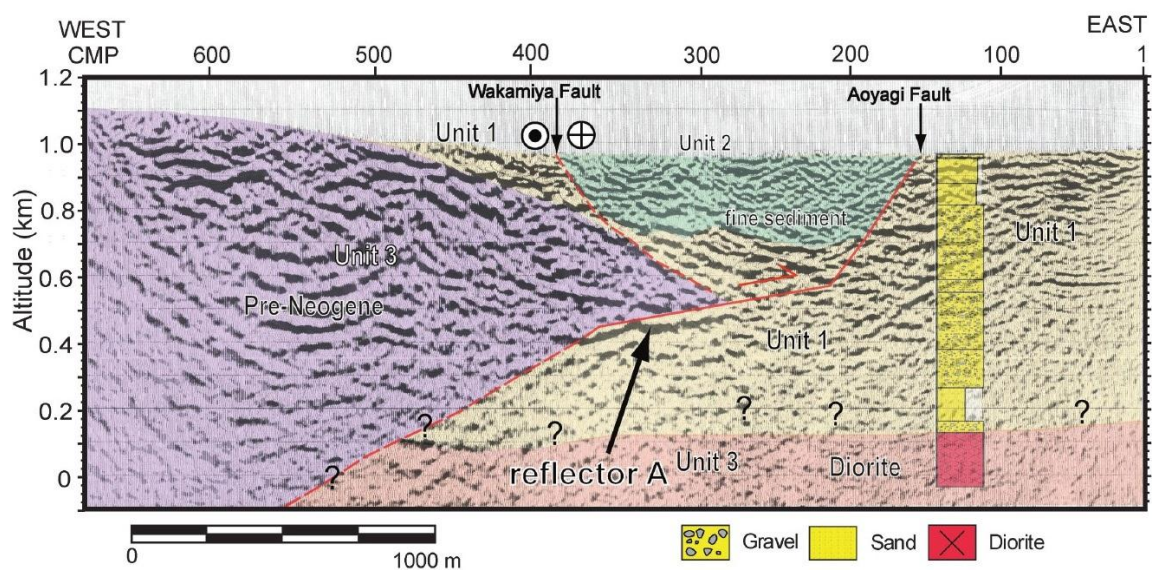
図4-4 浅層反射法地震探査（図2-3の測線F）の解釈図（松多ほか，2007b）
