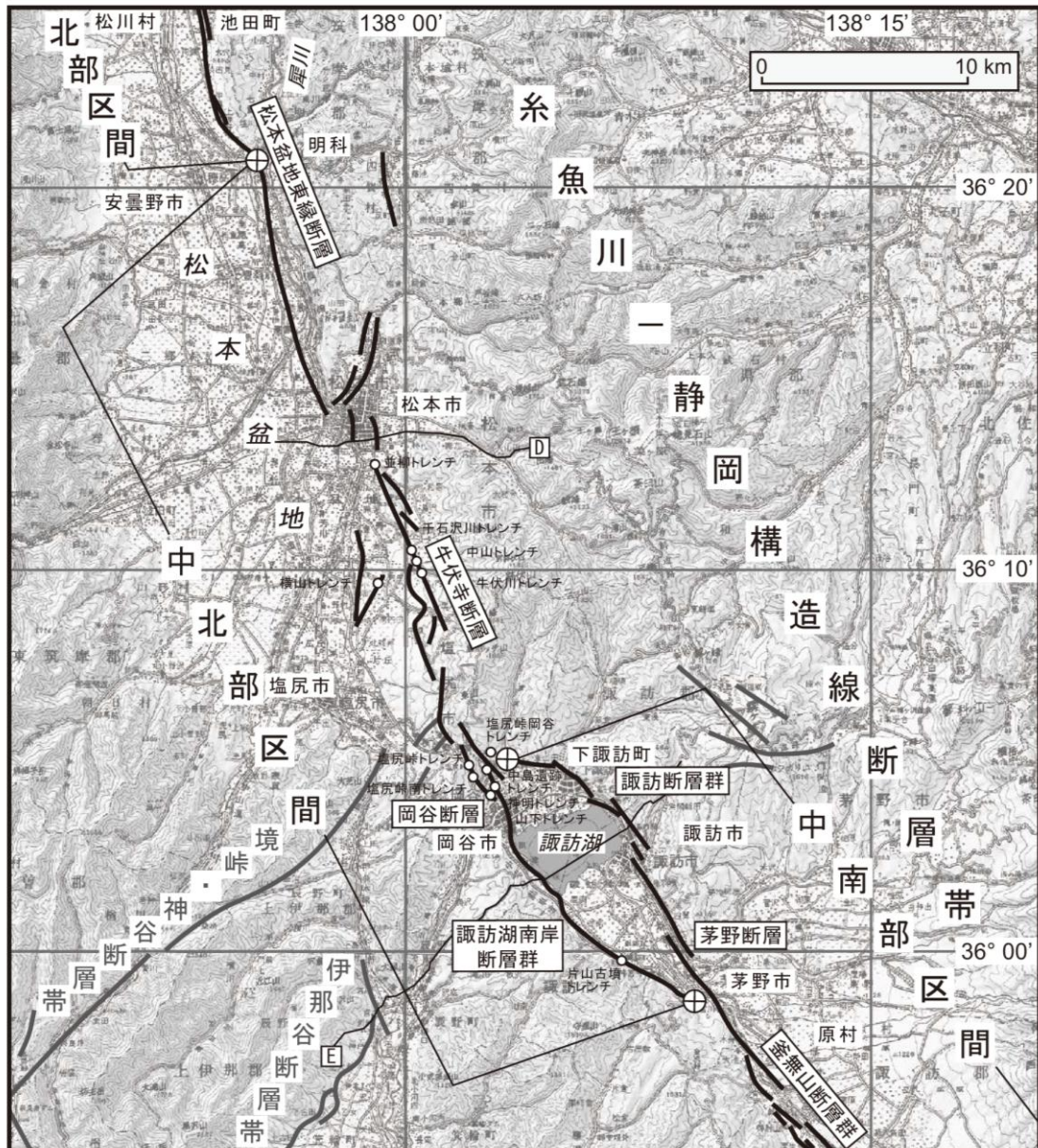
図 2-2 糸魚川—静岡構造線断層帯中北部（明科—諏訪湖南方）区間の活断層位置
