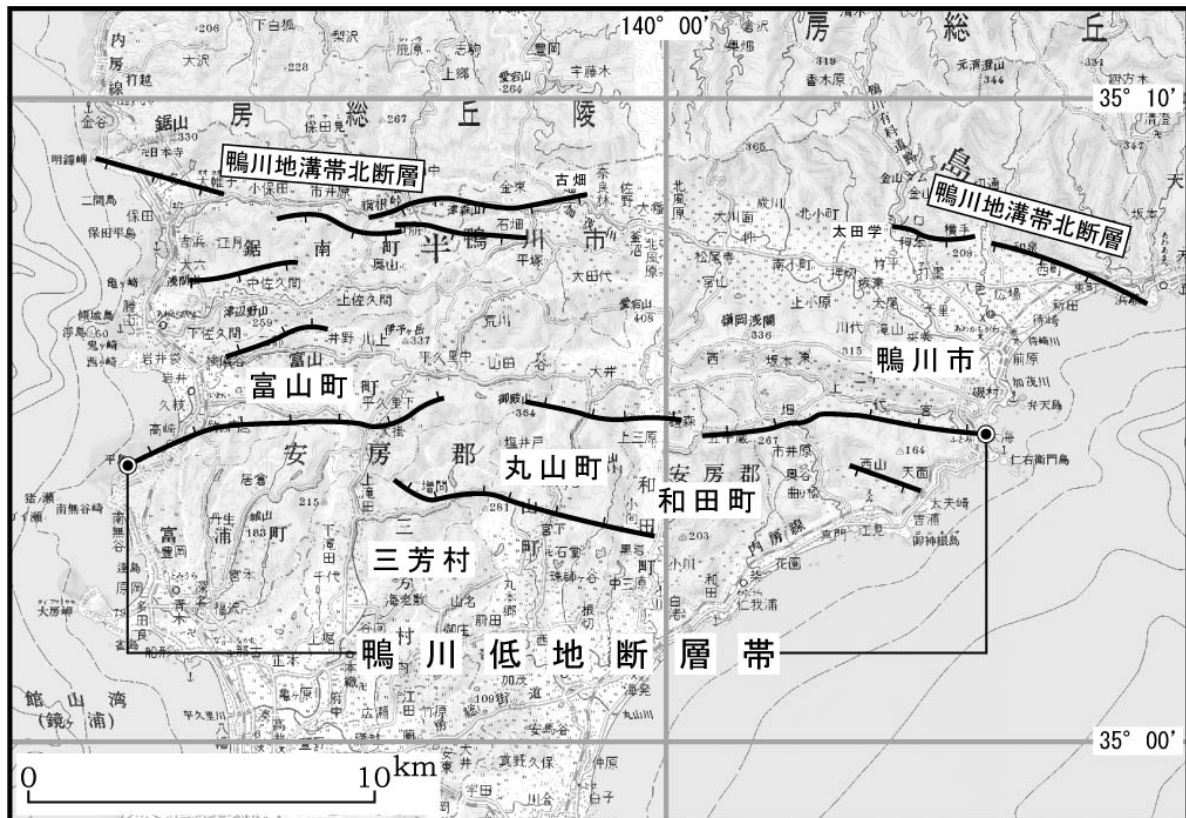
図3 鴨川低地断層帯の評価において考慮した断層
