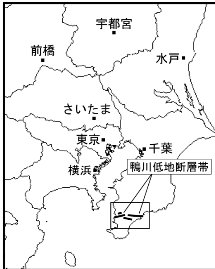
図1 鴨川低地断層帯の概略位置図 (長方形は図2の範囲)
