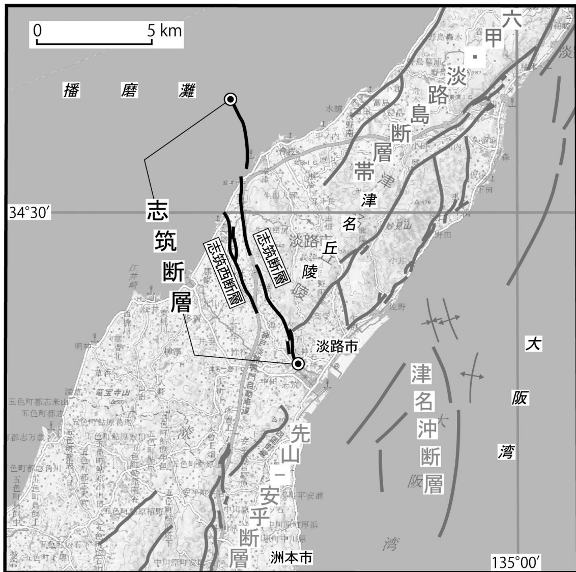
図1 志筑断層の位置
