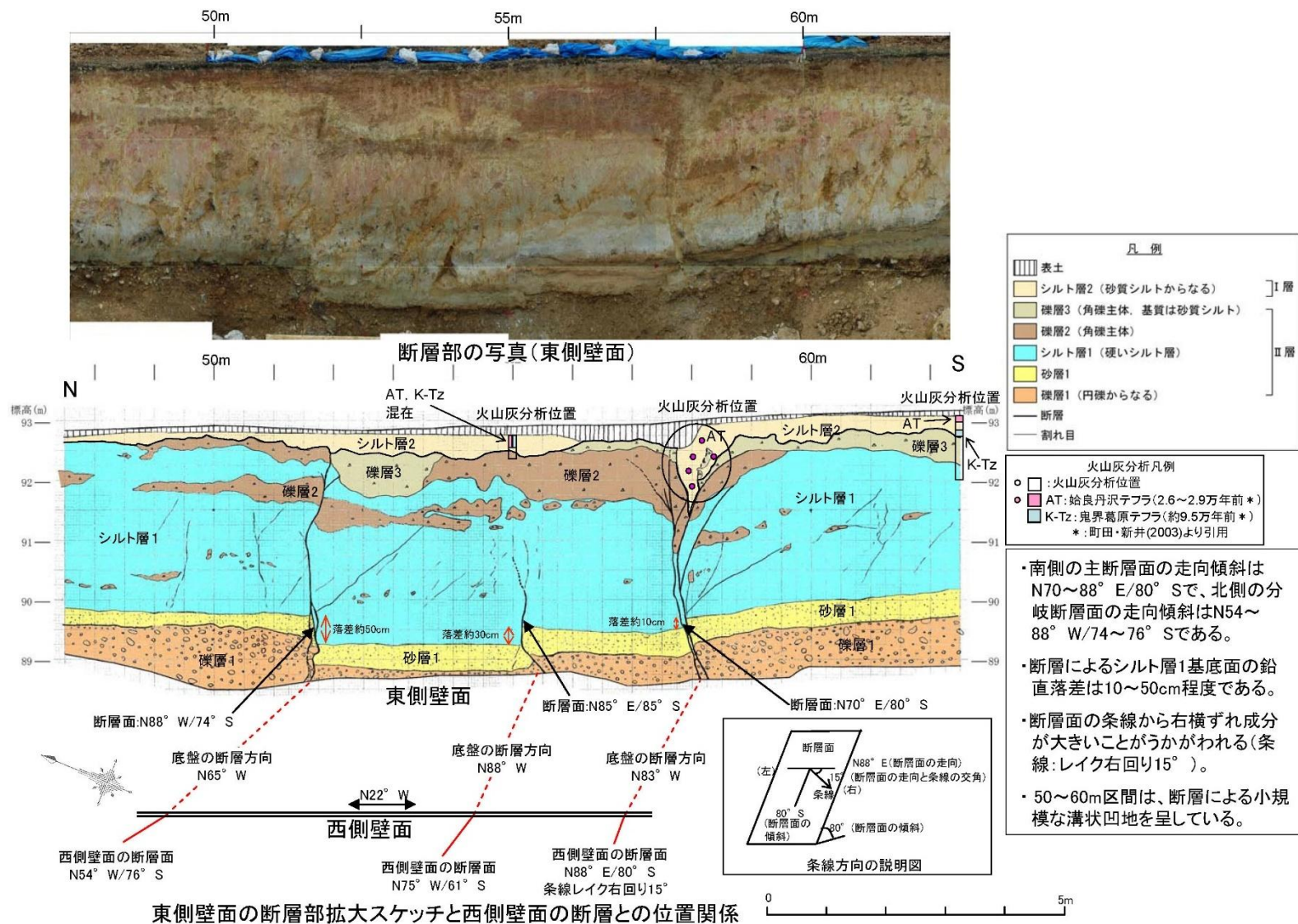
図4 上林川断層味方町地点におけるトレンチ壁面にみられる露頭スケッチ (関西電力, 2014) 始良 Tn (AT) 火山灰並びに鬼界葛原 (K-Tz) 火山灰を含む I 層が断層によって変位している。
