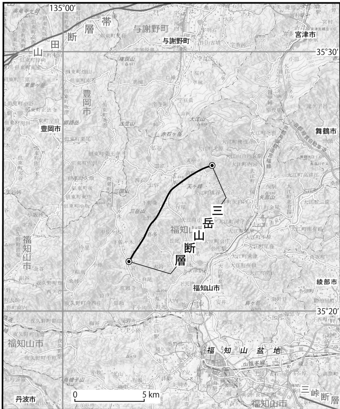
図1 三岳山断層の位置
