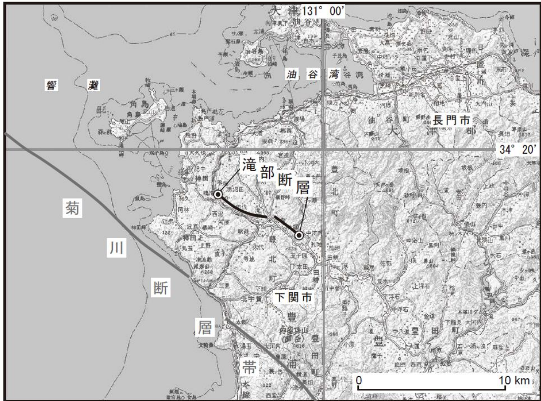
図1 滝部断層の位置
