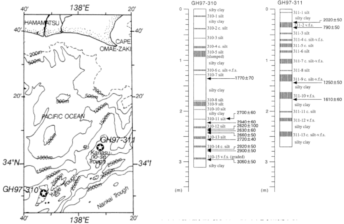
図 3-25 南海トラフ沿いにおけるタービダイトの採取地点（左）と研究対象試料の柱状図及び浮遊性有孔虫を用いた放射性炭素年代値（ \delta^{13}\text{C} 補正年代）（池原，2001） 柱状図でハッチをつけた部分がタービダイト、白抜き部は通常時に堆積した半遠洋性泥。
