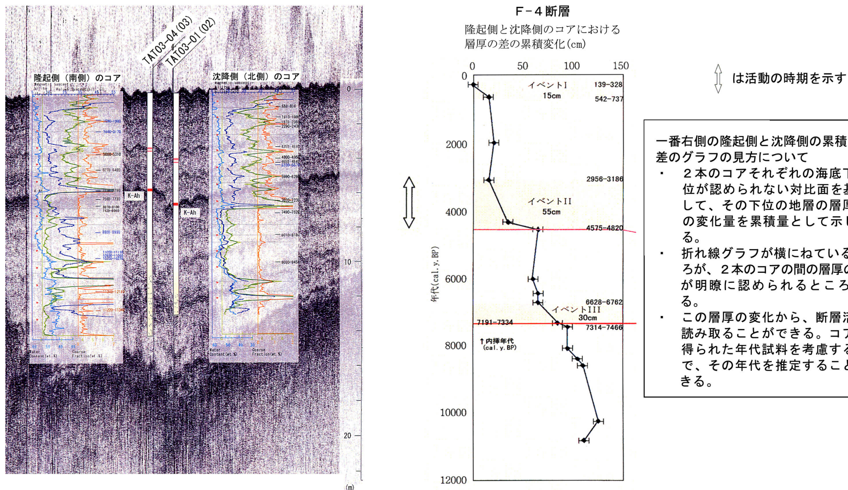
図4 F-4 断層有喜沖南方沖地点における音波探査結果とコア解析 長崎県 (2004) に一部加筆・修正
