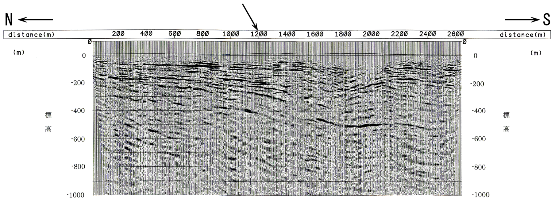
図3 島原市内における反射法地震探査断面 長崎県（2005）に断層の位置を加筆
