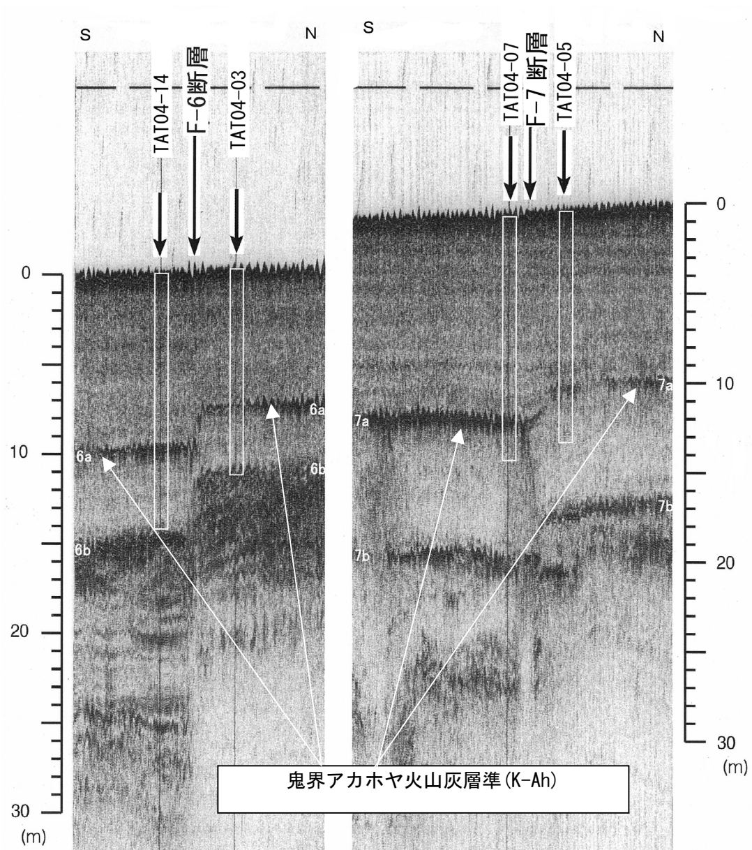
図 10 F-6・F-7 断層の音波探査結果 長崎県 (2005)
