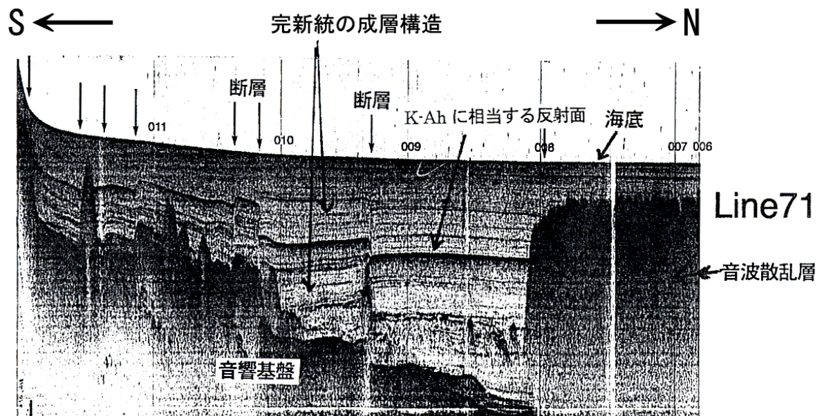
図8 F-1 から F-3 断層にほぼ直交する音波探査結果 (長崎県, 2003)
