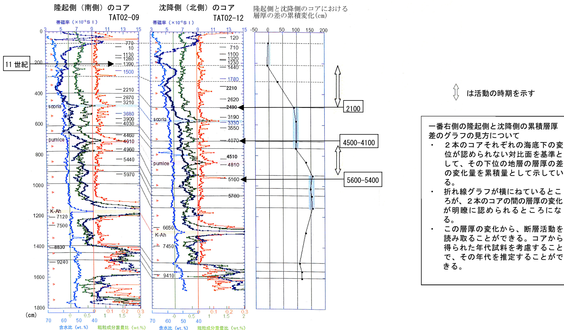
図9 F-3断層小浜—金浜沖地点におけるコア解析 長崎県（2003）に一部加筆
