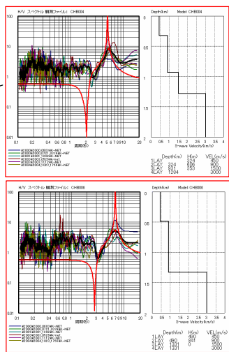
地震観測記録と 計算波形のH/V スペクトル比 田中・他 (2005)
