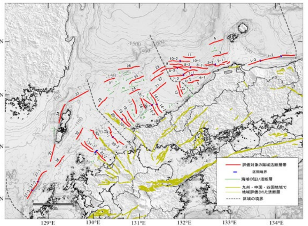
日本海南西部(評価対象海域)における評価対象の海域活断層帯と海域の短い活断層の分布
