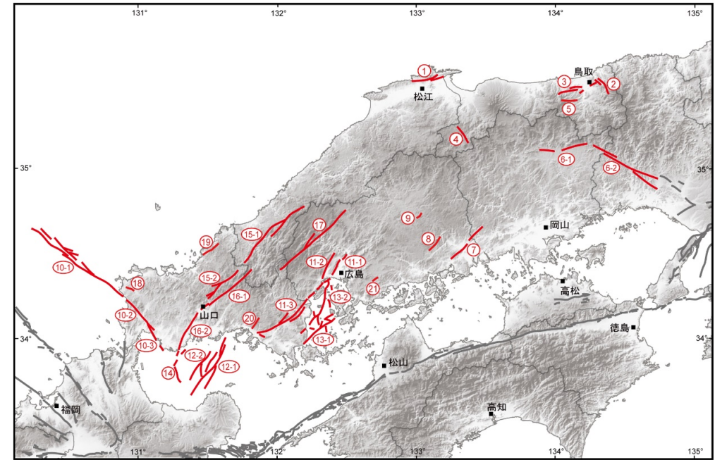
中国地域（評価対象地域）において評価対象とした活断層の分布
