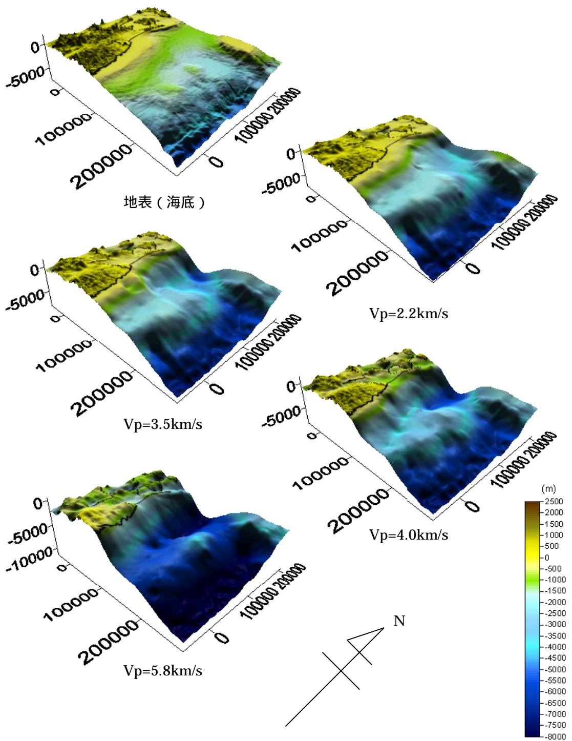
図3 深い地盤構造モデル鳥瞰図 (日本平面直角座標第 系)
