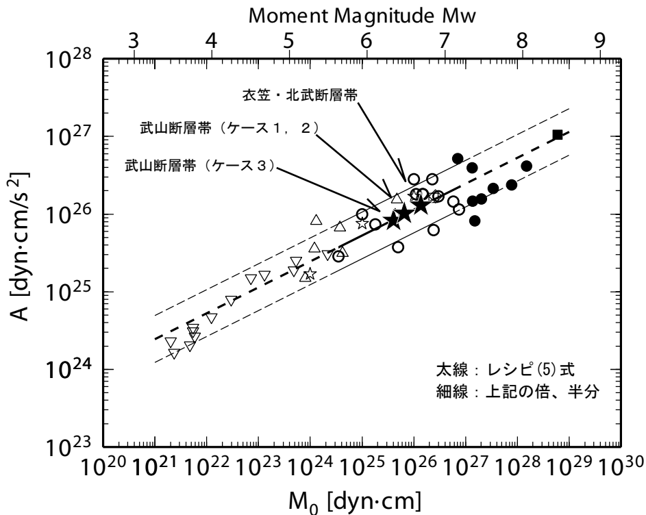
図10 地震モーメント M_0 と断層面積 S の経験的關係(上)および地震モーメント M_0 と短周期レベル A の経験的關係(下)
